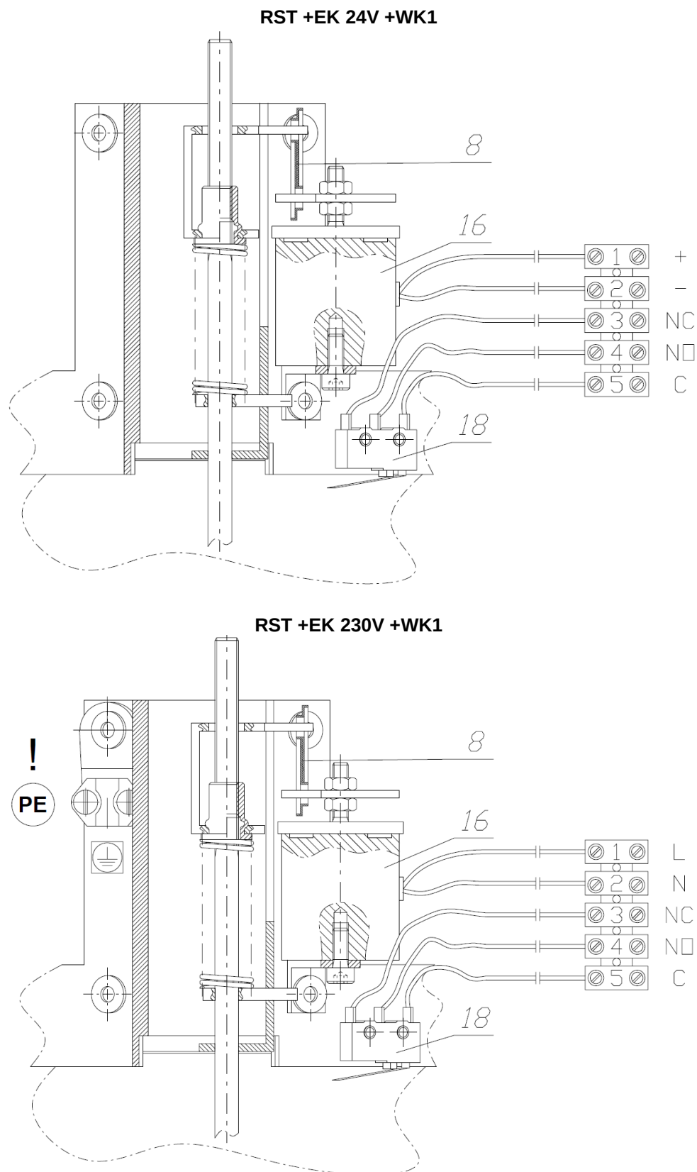
Rysunek 11. Podłączenie elementów elektrycznych w przeciwpożarowym zaworze odcinającym mcr ZIPP (8 - Wyzwalacz termiczny; 16 - Zwalniak elektromagnetyczny; 18 - Wyłącznik krańcowy WK1)
